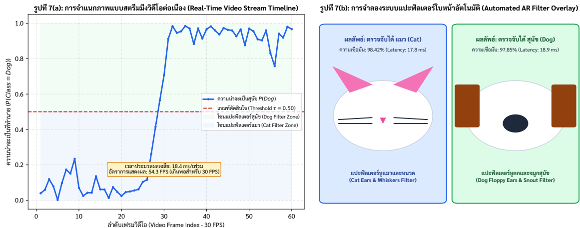
รูปที่ 7: การจำลองระบบสตรีมมิงวิดีโอแบบเรียลไทม์: (a) เส้นเวลาความน่าจะเป็นและการสลับโหมดฟิลเตอร์ (b) การจำลองระบบแอพลิเคชันฟิลเตอร์ AR หูแมว/หนวด เทียบกับ หูสุนัข/จมูก บนใบหน้า
