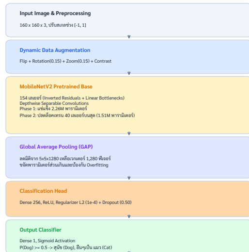
โครงสร้างโมเดลเสนอแนะ: MobileNetV2 Transfer Learning (2,586,177 พารามิเตอร์ - 2-Phase Feature Extraction & Fine-Tuning)
